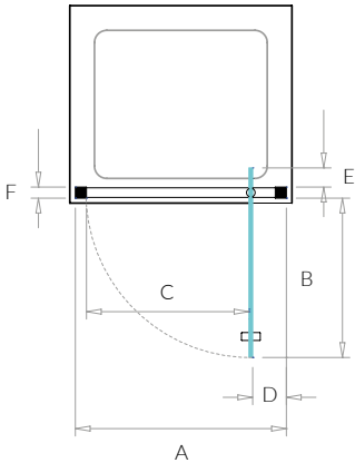
Pivot Door Diagram
